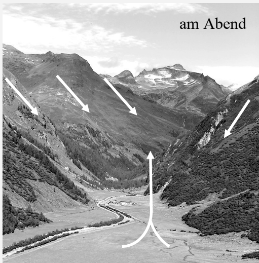
Kaltluft sinkt ins Tal, Umkehrthermik wird ausgelöst.
