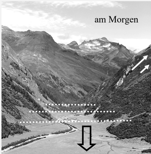
Der Kaltluftsee wird abgebaut. Erste Thermik entwickelt sich.
