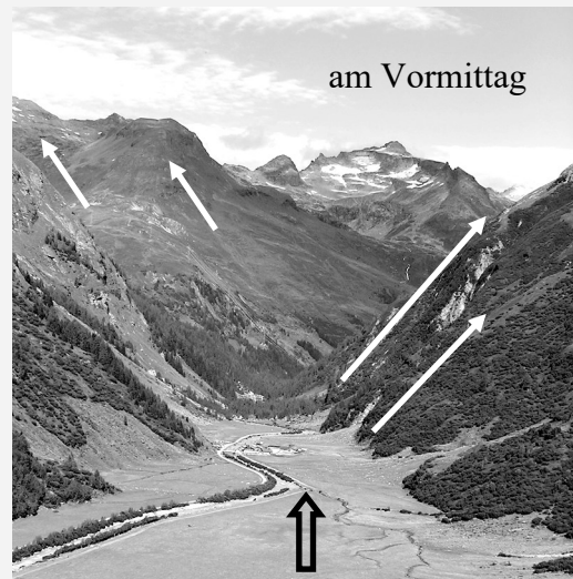
Der Talwind kommt zum Stillstand. Der Bergwind entwickelt sich.
